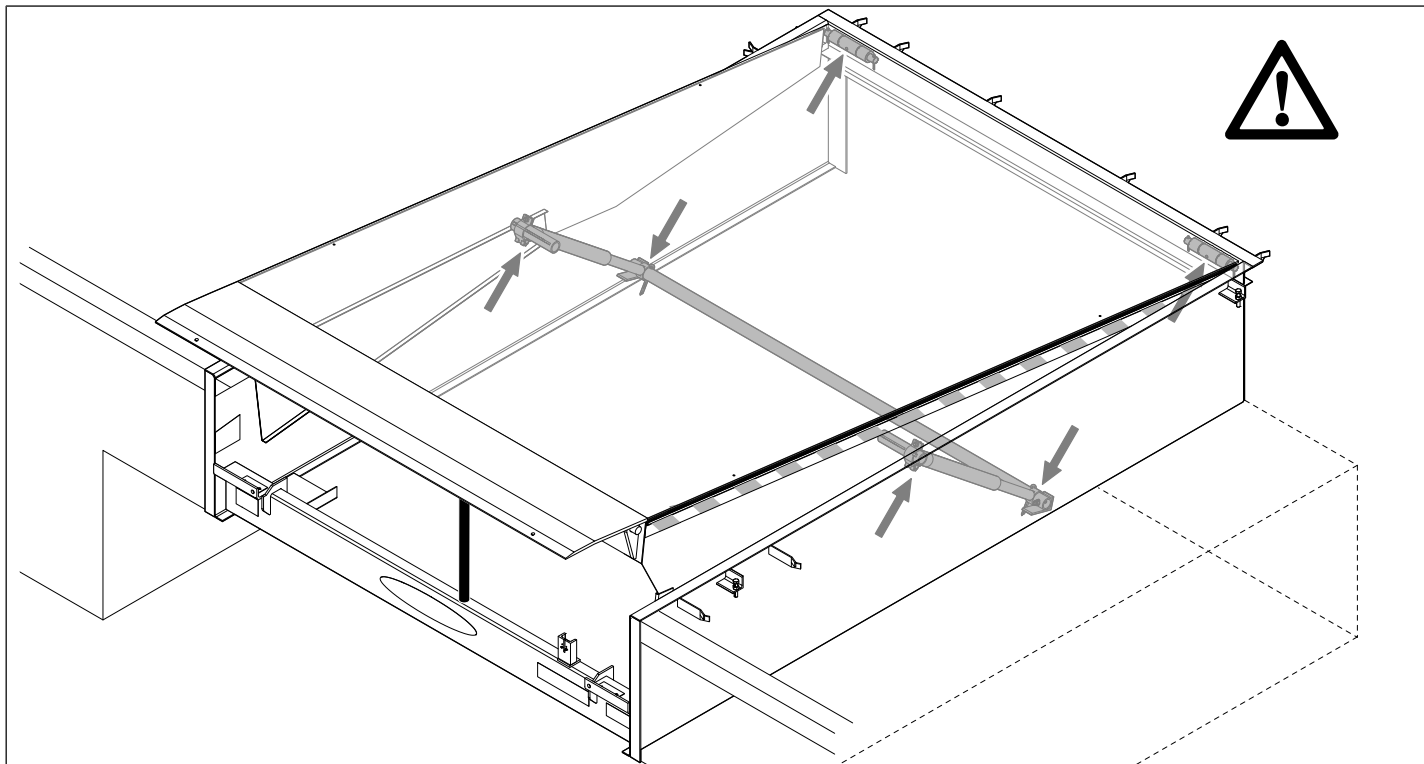
Fig. 7: Puntos de engrase, la imagen puede diferir del producto
