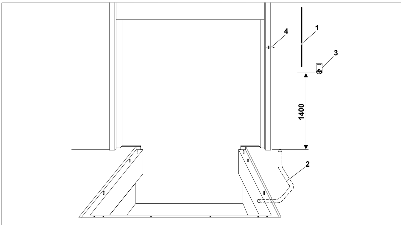
Abb. 6: Exemplarische Darstellung für Einbausituation CZ
