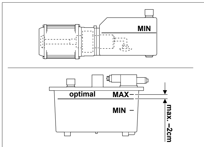
Fig. 8: Nível de óleo
