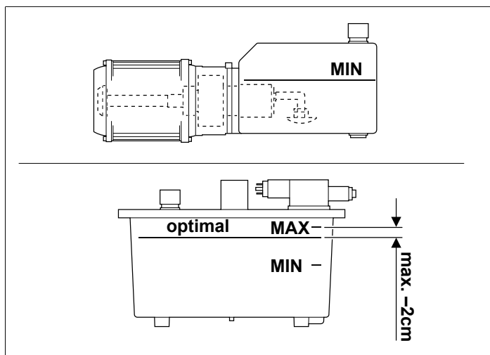
Fig. 8: Niveau d'huile
