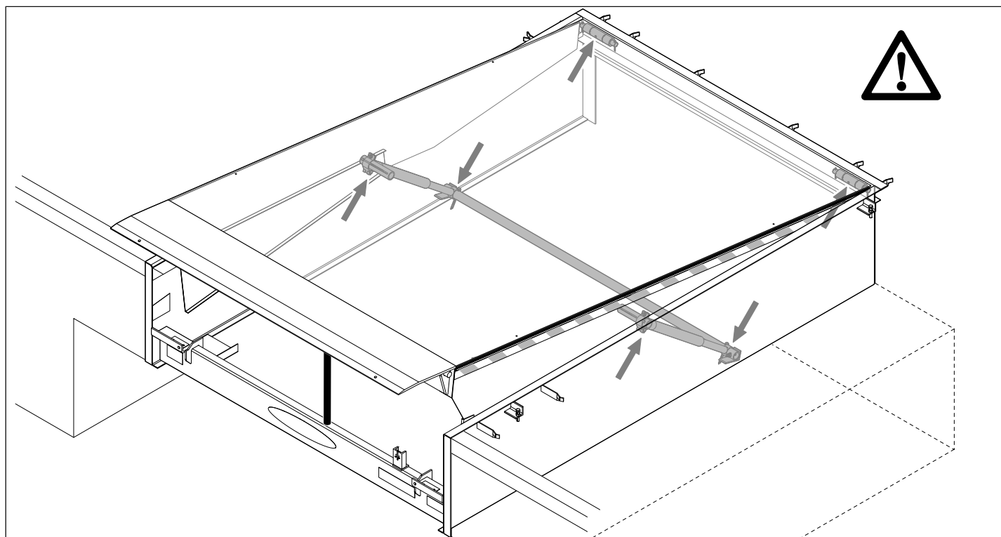
Abb. 7: Schmierstellen, Abbildung kann vom Produkt abweichen
