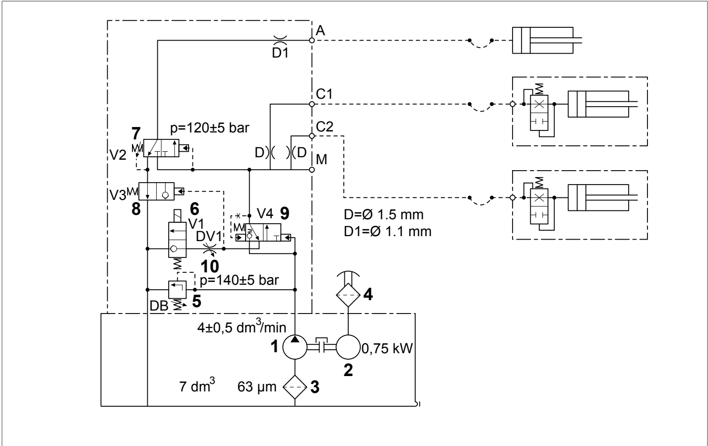
Fig. 5: Schéma hydraulique
