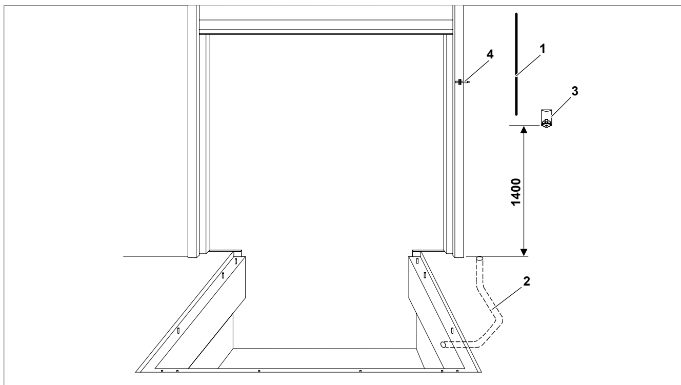
Afb. 6: Voorbeeldweergave voor inbouwsituatie CZ
