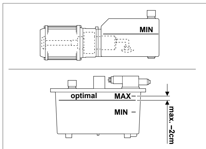
Afb. 8: Oliepeil
