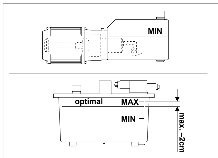
Fig. 8: Nivel de aceite
