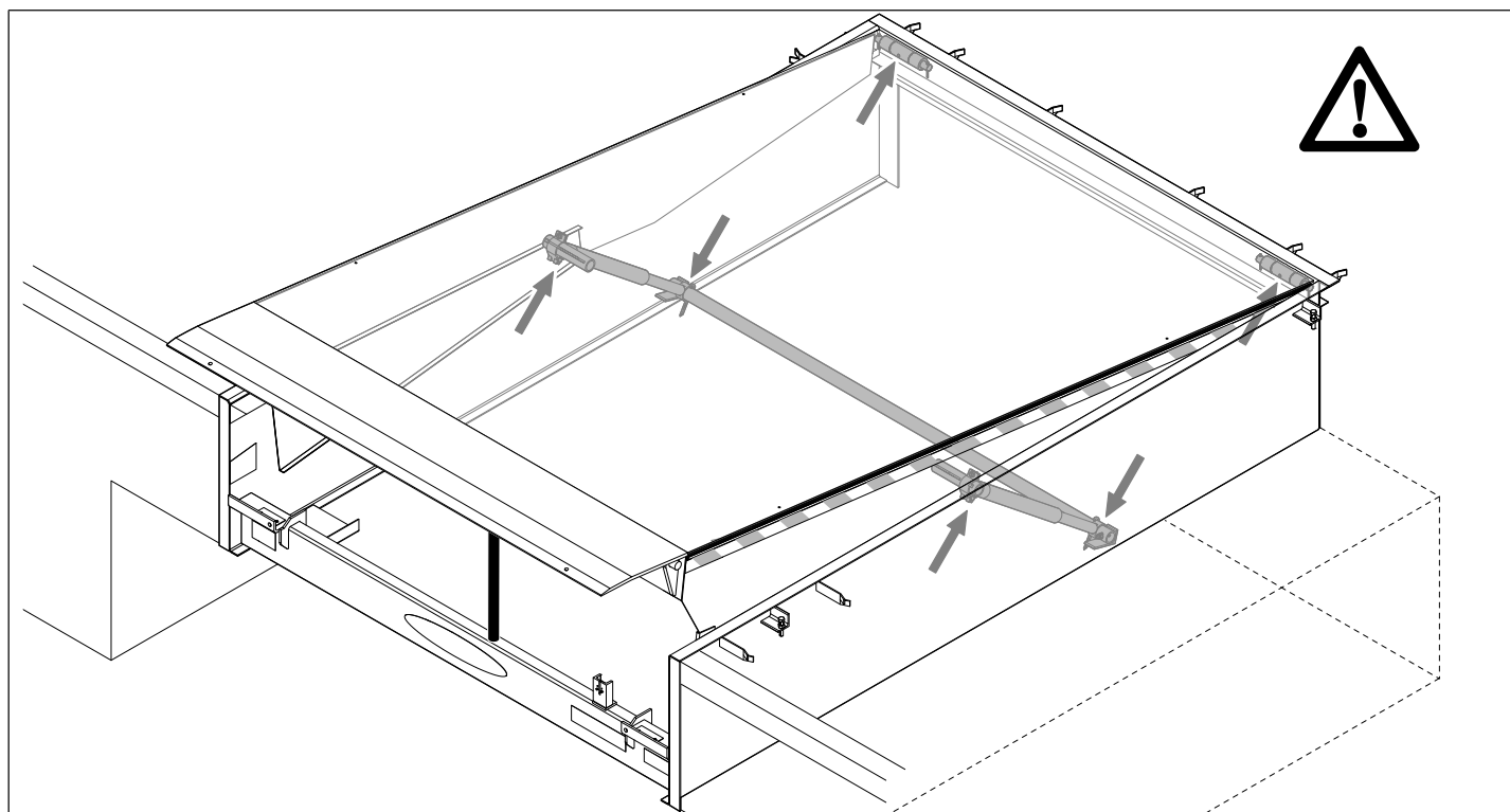
Fig. 7: Pontos de lubrificação, a figura pode divergir do produto
