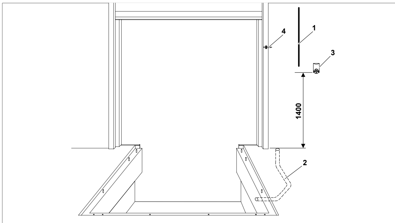
Fig. 6: Imagem exemplar para a situação de montagem CZ
