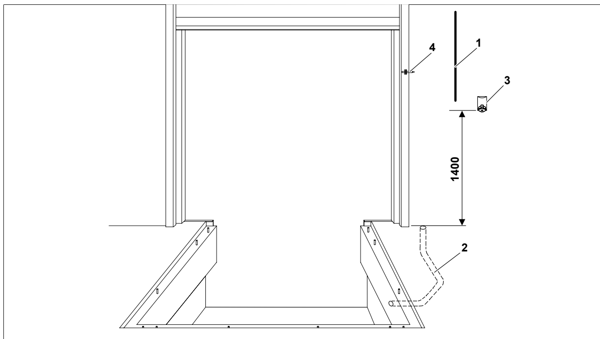
Fig. 6: variante de montage CZ (exemple)
