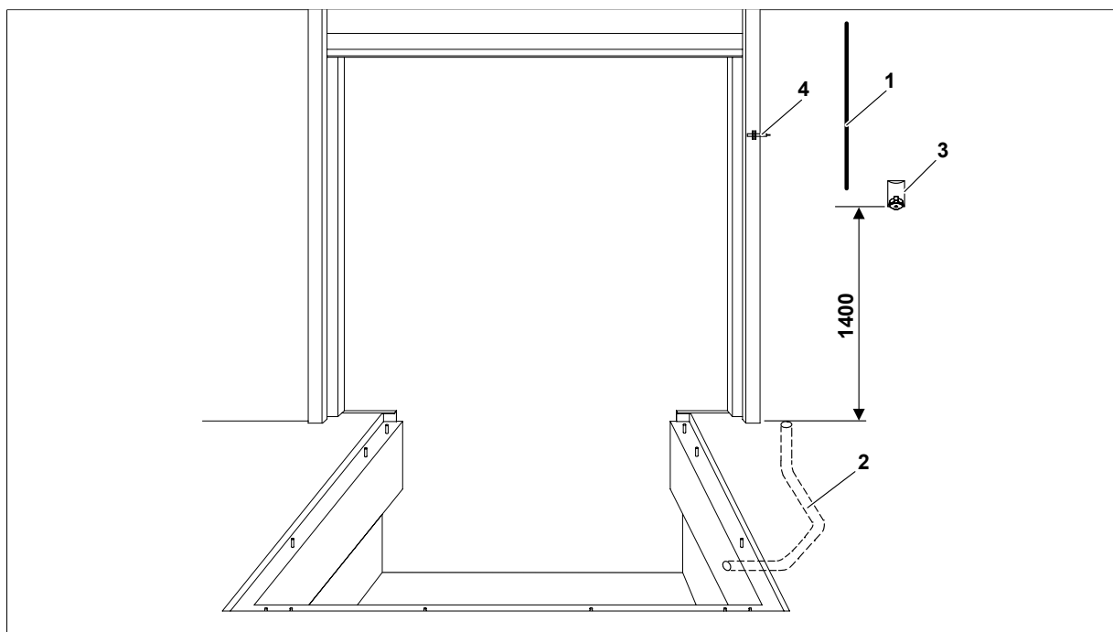
Fig. 6: Representación a modo de ejemplo para la situación de instalación CZ
